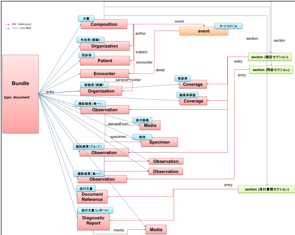
図1 文書構造の概要 (FHIR リソースで構造化する場合)
